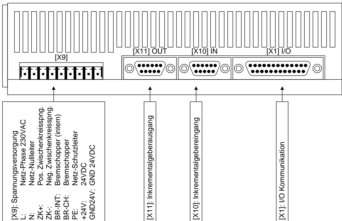
Abbildung 5: Servopositionierer SE-Power FS 1kVA: Ansicht oben
