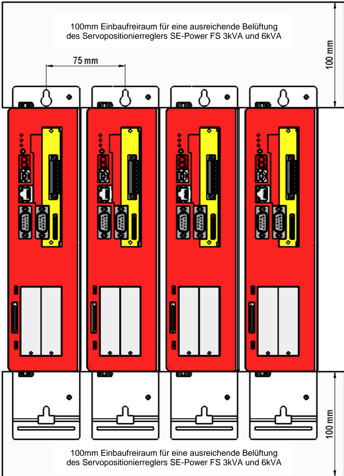
Abbildung 2: Servopositionierregler SE-Power FS 3kVA und 6kVA: Einbaufreiraum
