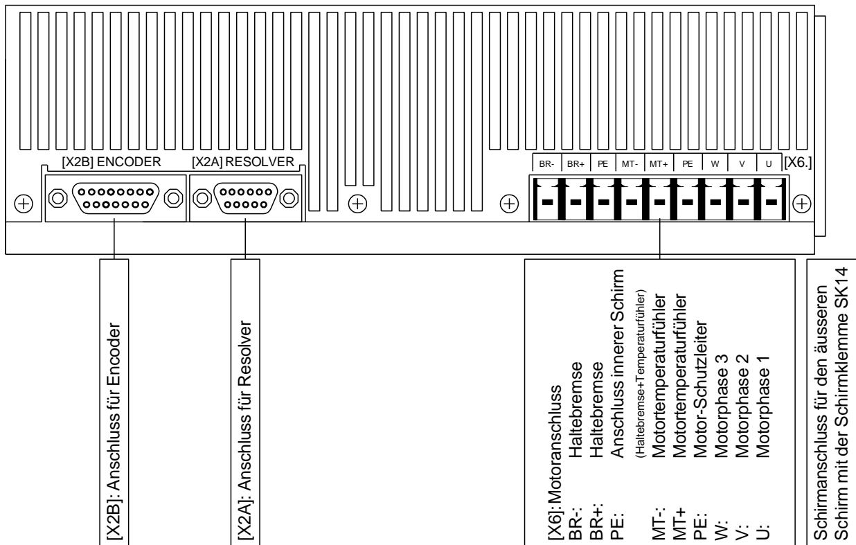
Abbildung 8: Servopositionierregler SE-Power FS 3kVA und 6kVA: Ansicht unten
