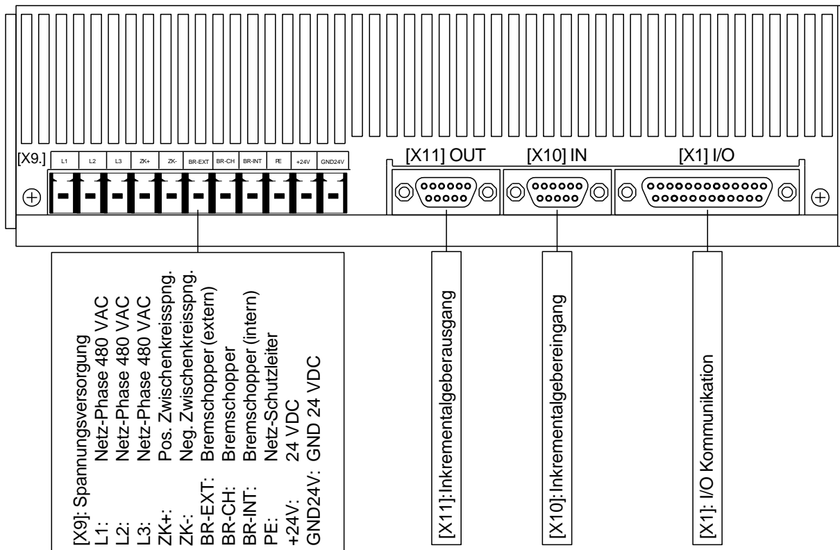
Abbildung 7: Servopositionierregler SE-Power FS 3kVA und 6kVA: Ansicht oben
