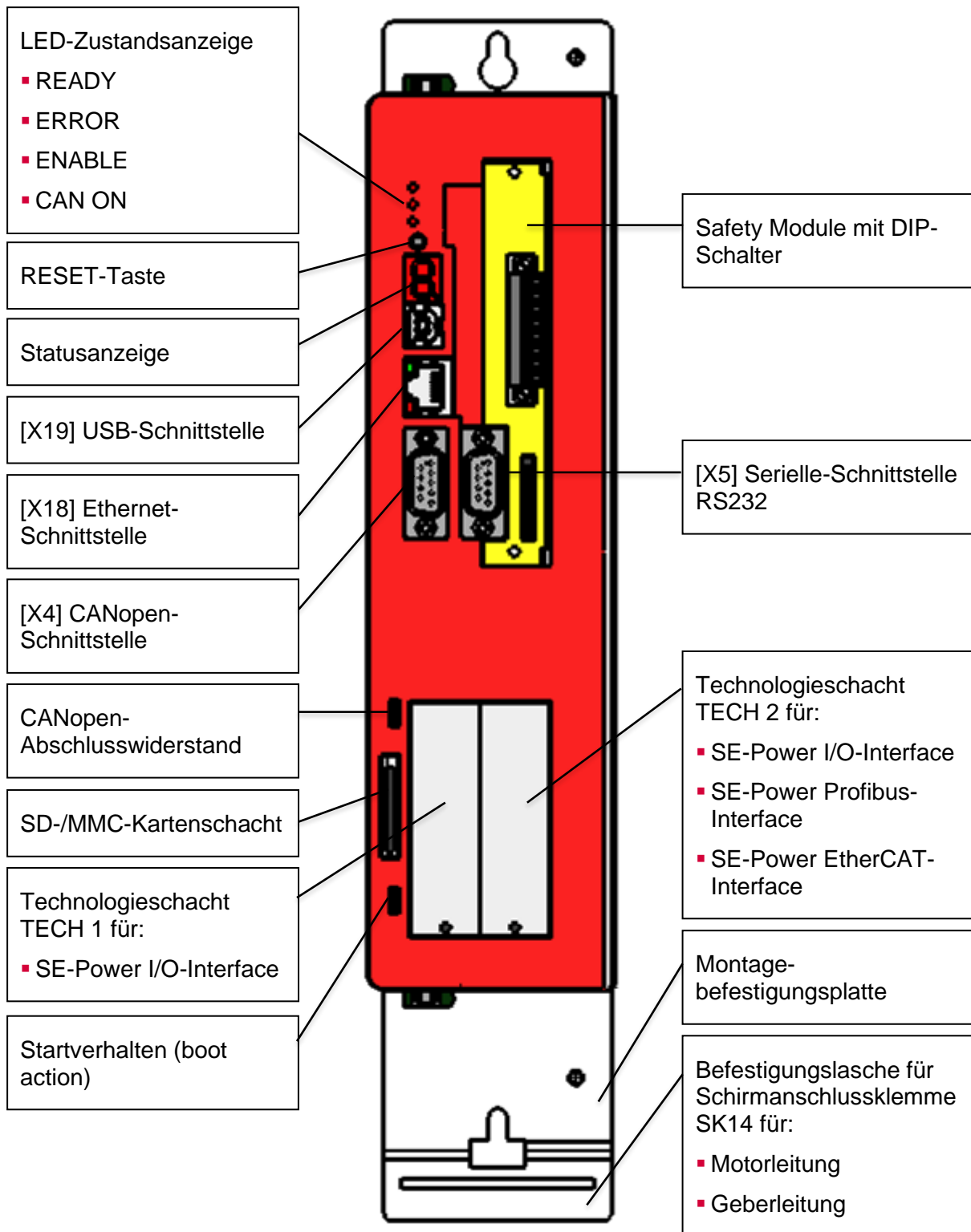
Abbildung 4: Servopositionierregler SE-Power FS 3kVA und 6kVA: Ansicht vorne
