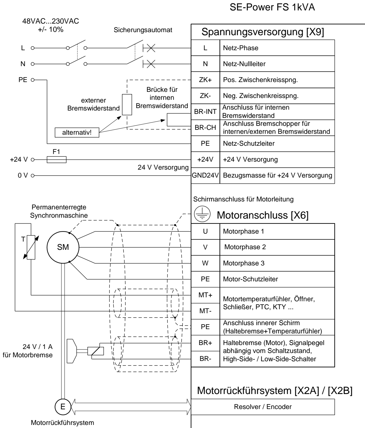
Abbildung 11: Anschluss SE-Power FS 1kVA an die Versorgungsspannung und den Motor
