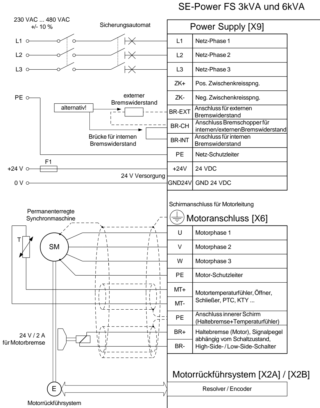
Abbildung 12: Anschluss SE-Power FS 3kVA und 6kVA an Versorgungsspannung und Motor
