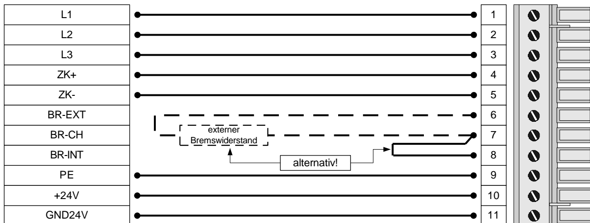
Abbildung 14: Versorgung [X9] SE-Power FS 3kVA und 6kVA
