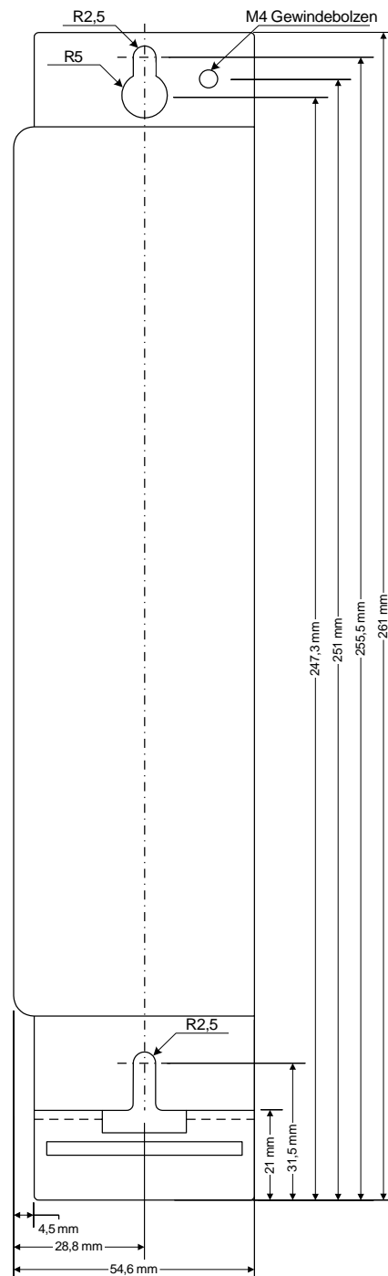
Abbildung 9: Servopositionierregler SE-Power FS 1kVA: Befestigungsplatte
