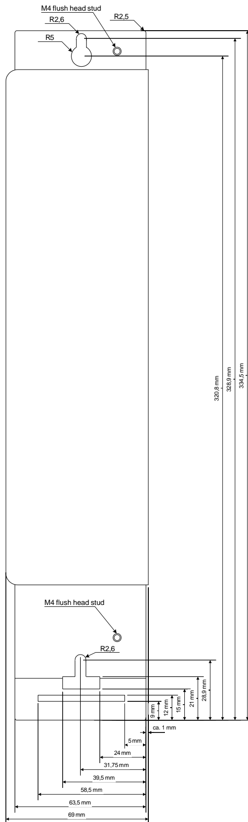
Abbildung 10: Servopositionierregler SE-Power FS 3kVA und 6kVA: Befestigungsplatte
