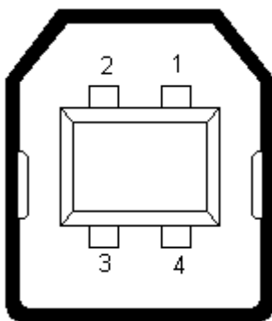
Abbildung 16: Pinbelegung: USB-Schnittstelle [X19], Frontansicht
