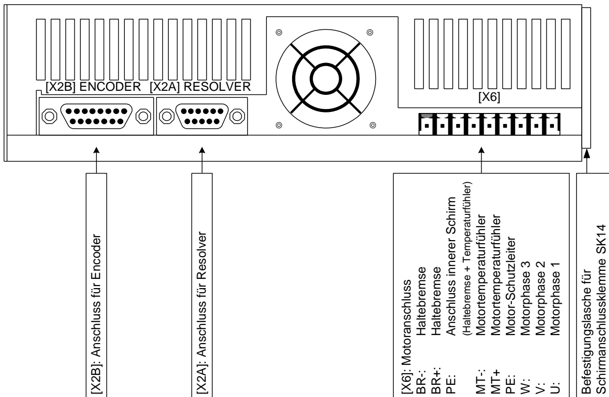
Abbildung 6: Servopositionierer SE-Power FS 1kVA: Ansicht unten
