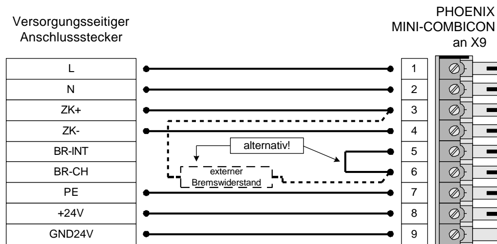
Abbildung 13: Versorgung [X9] SE-Power FS 1kVA
