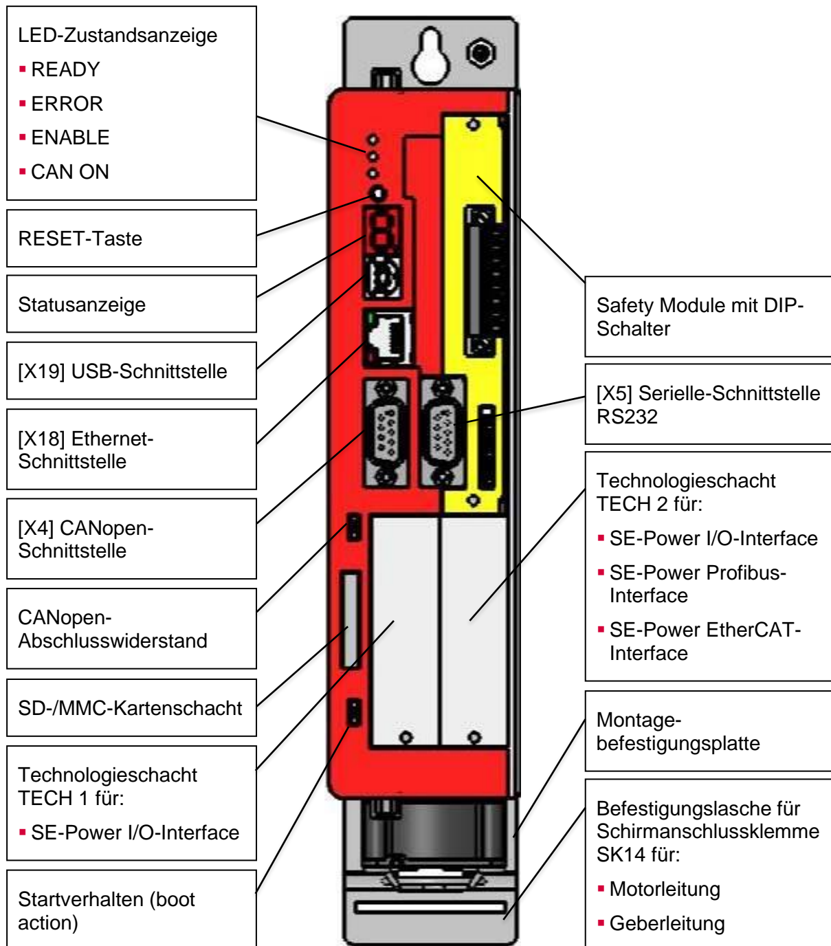
Abbildung 3: Servopositioniererregler SE-Power FS 1kVA : Ansicht vorne
