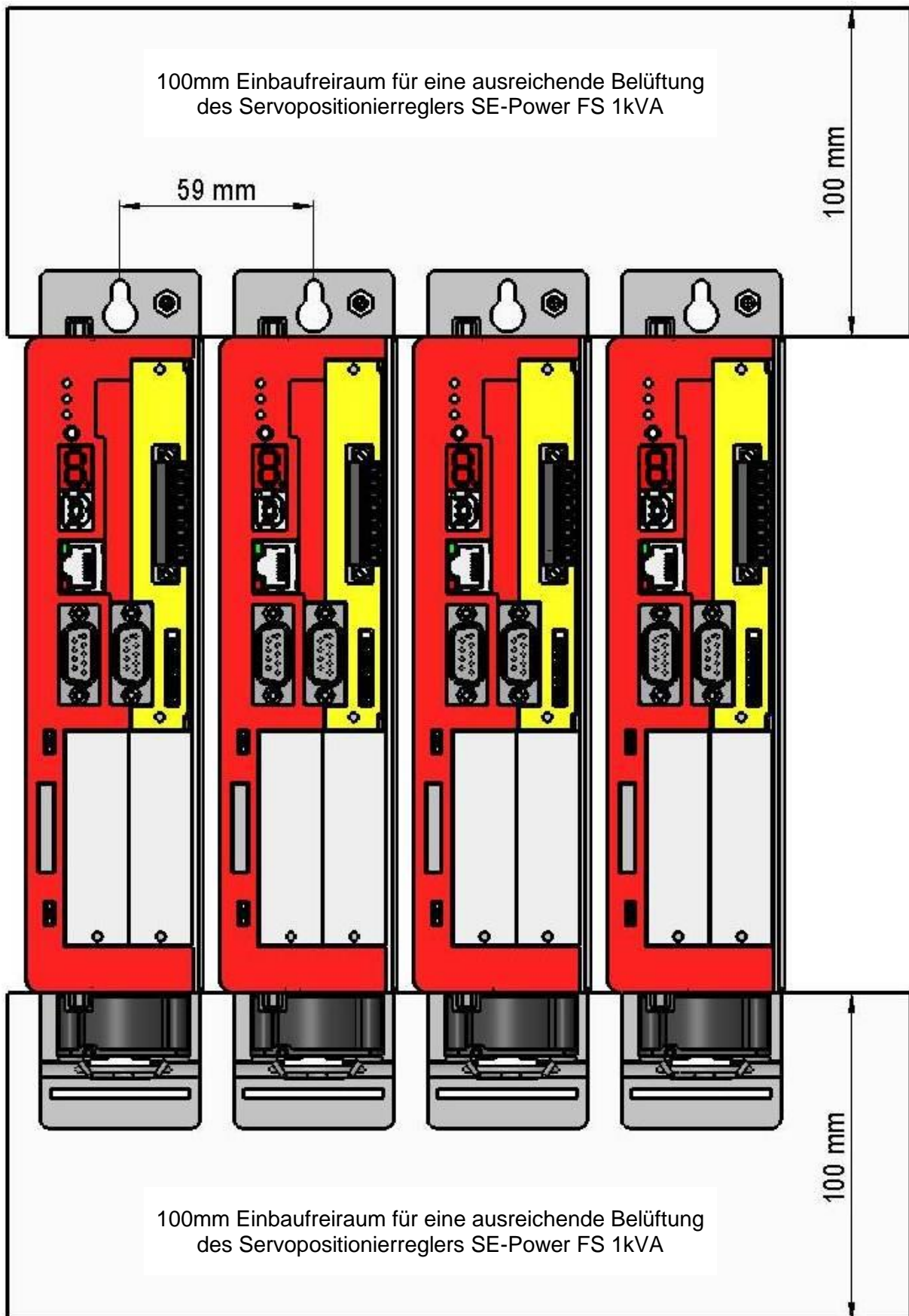
Abbildung 1: Servopositionierregler SE-Power FS 1kVA: Einbaufreiraum
