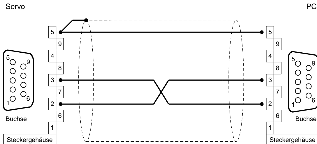
Abbildung 15: Steckerbelegung RS232-Nullmodemkabel [X5]
