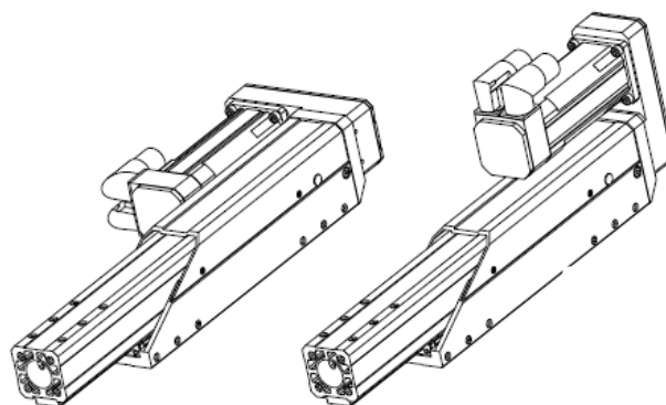
Fig. 5 Positions du servomoteur
