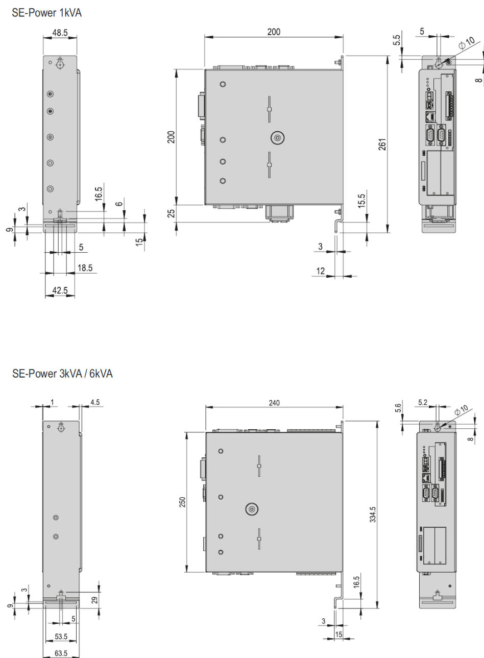
Fig. 10 Installation - SE-Power pour montage en armoire électrique
