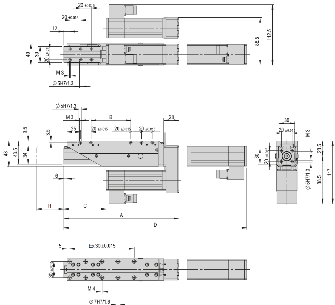
Fig. 1 Dessin coté axe télescopique
