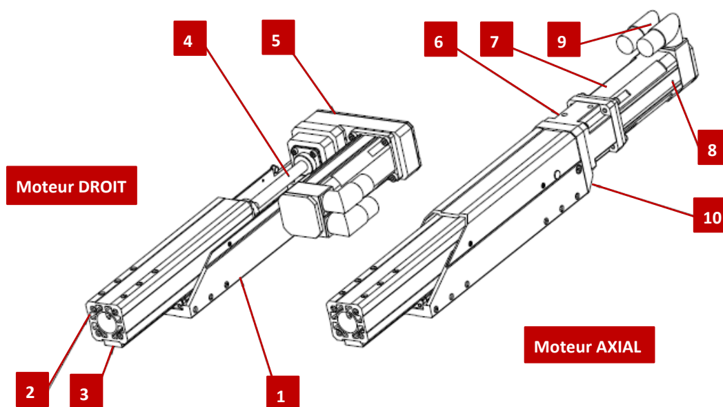
Fig. 6 Montage du moteur DROIT / AXIAL
