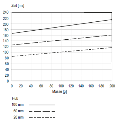
Abb. 2 Belastungen Elektroschlitten
