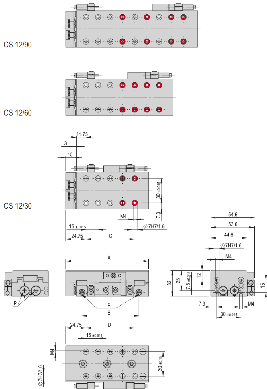
Abb. 5 Masszeichnung Compact-Schlitten CS 12
