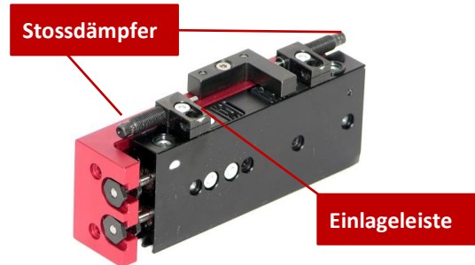
Abb. 16 Einstellung der Stossdämpfer
