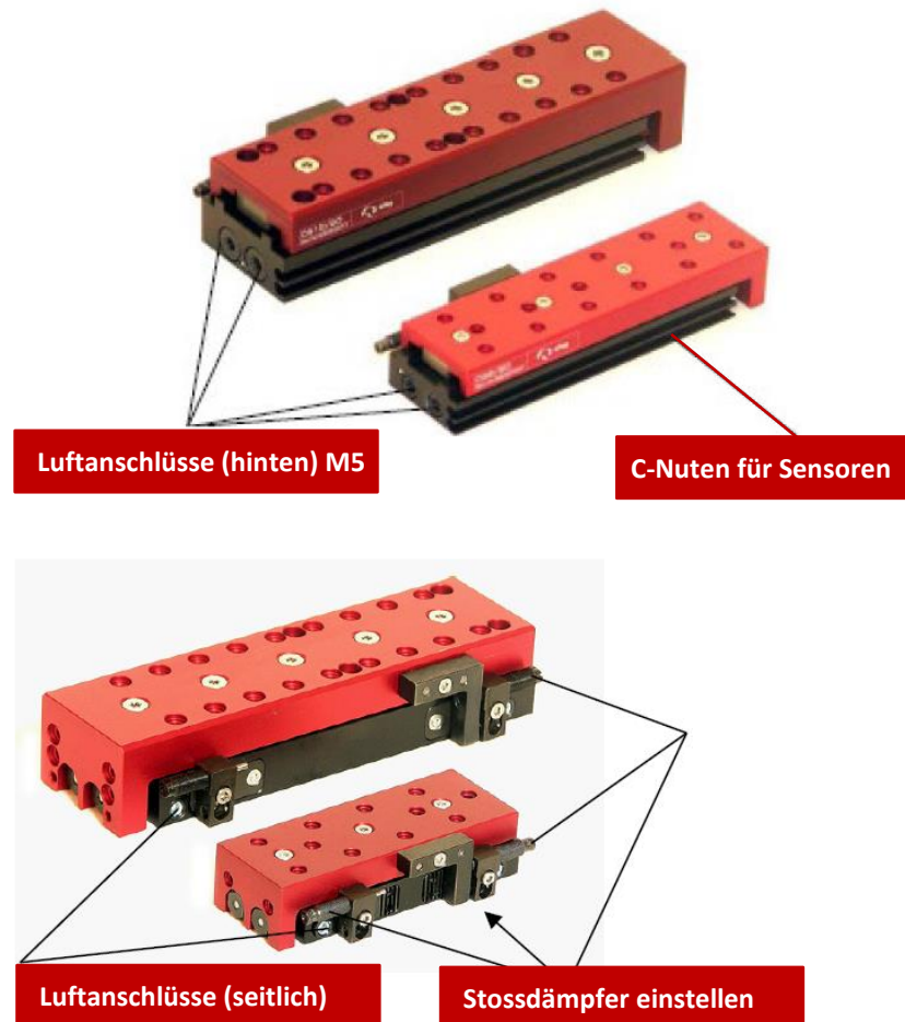
Abb. 17 Einstellung der Hydraulik-Stossdämpfer
