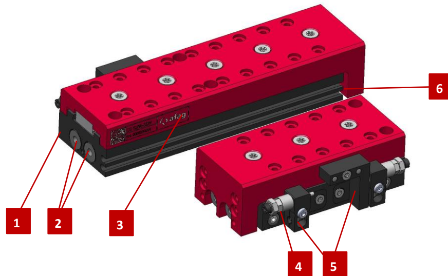
Abb. 10 Aufbau des CS Moduls
