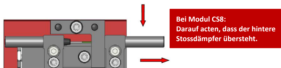
Abb. 17 Einstellung der Hydraulik-Stossdämpfer
