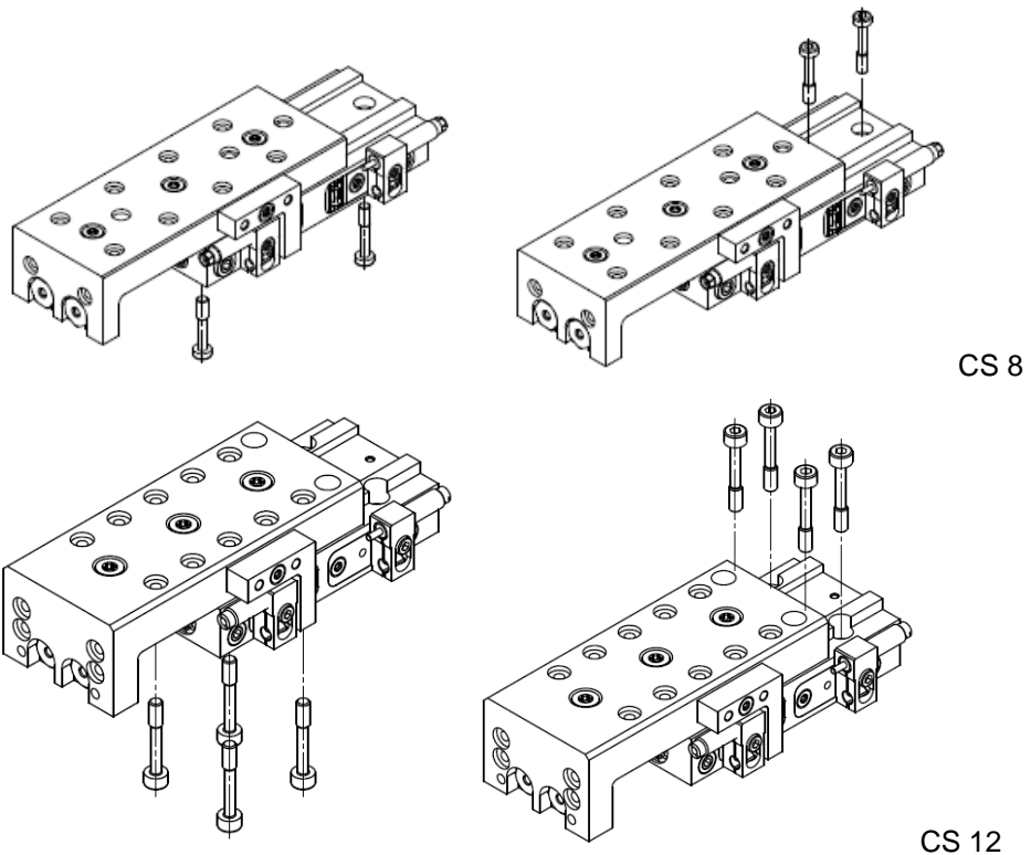
Abb. 11 Montage Grundkörper von unten Montage Grundkörper durchgeschraubt
