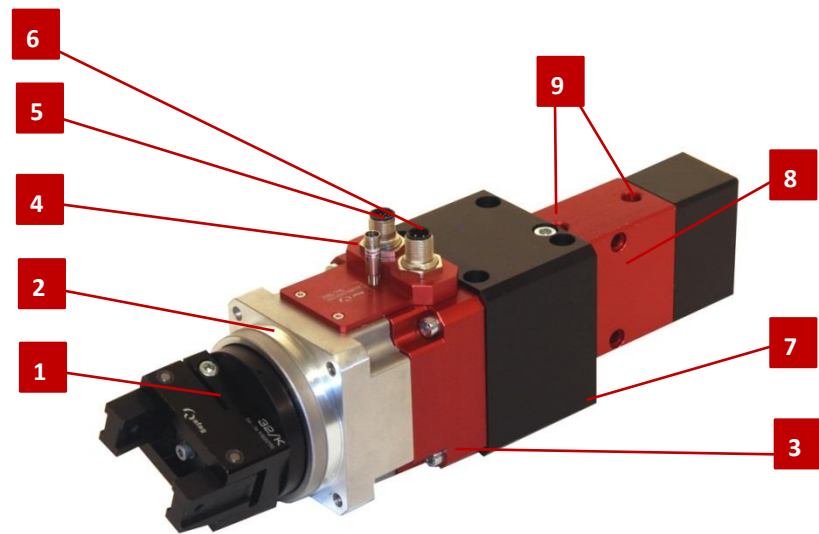
Abb. 8 Greif-Drehmodul pneumatisch-elektrisch
