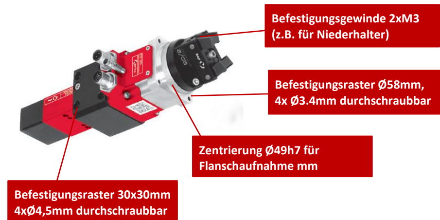
Abb. 5 Befestigung Greif-Drehmodule
