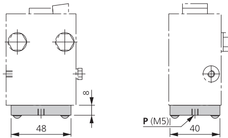
P = Luftanschluss / Raccordement d'air / Air connection
