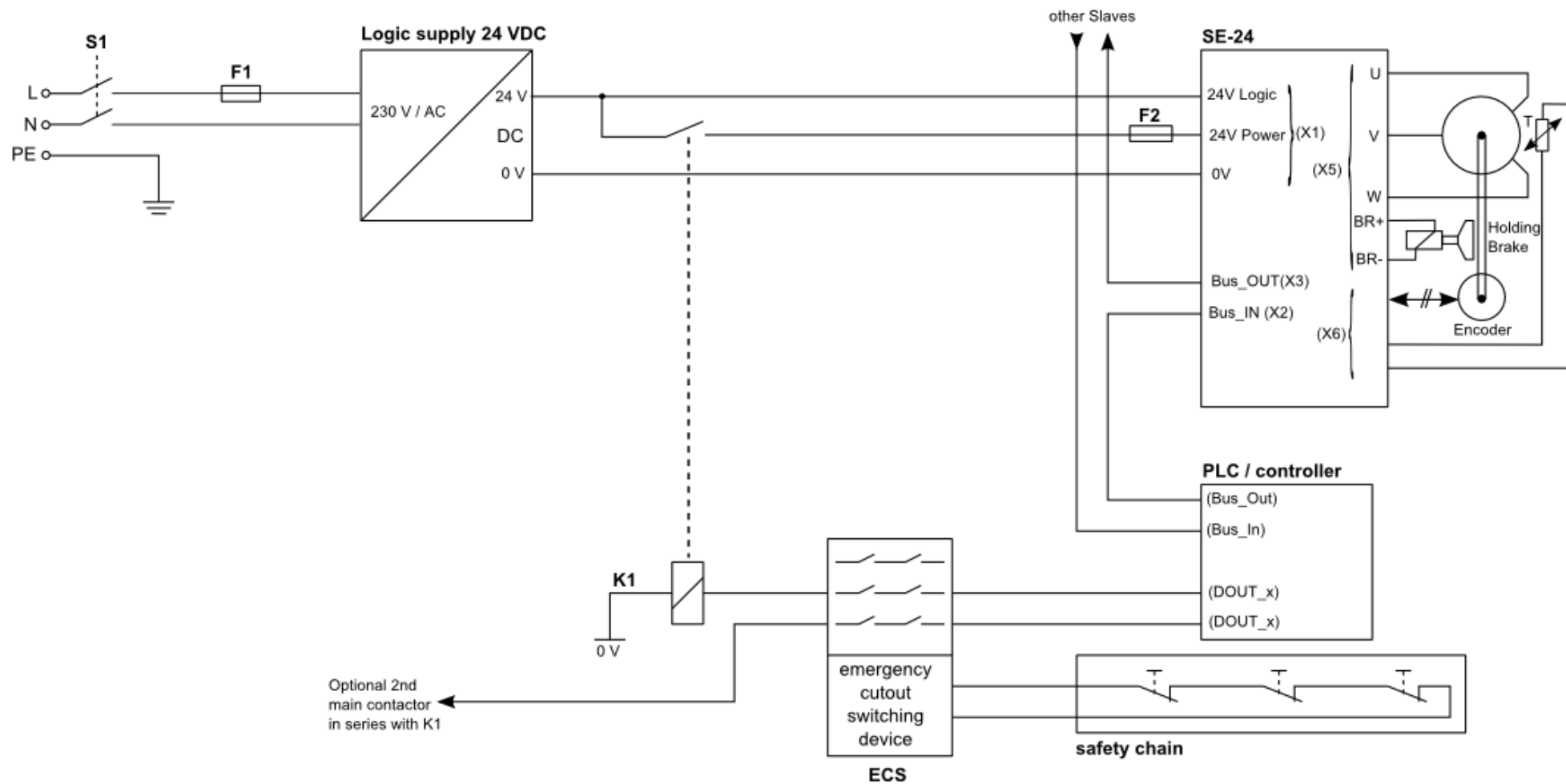
Figure 18: Câblage-type du bus de terrain du SE-24
