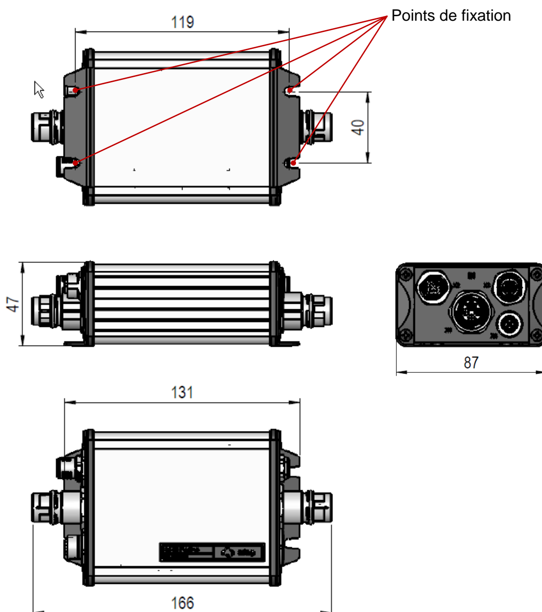
Figure 2: Dimensions et points de fixation
