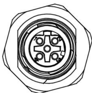
Figure 9: Vue des branchements [X3d]
